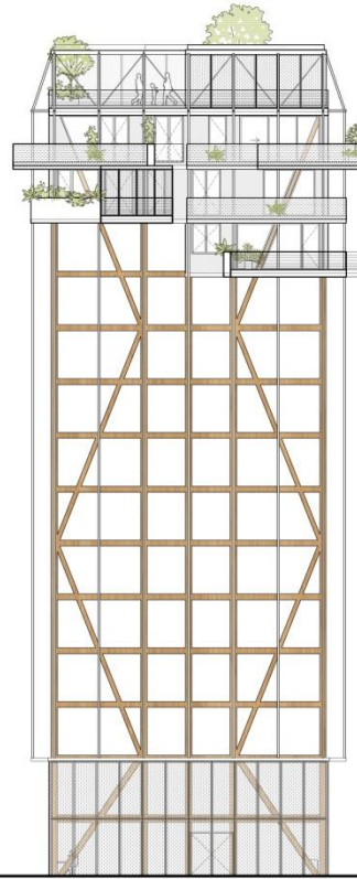
Façade Sud-Ouest
