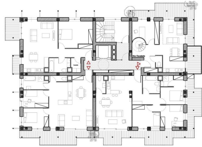
R+2
