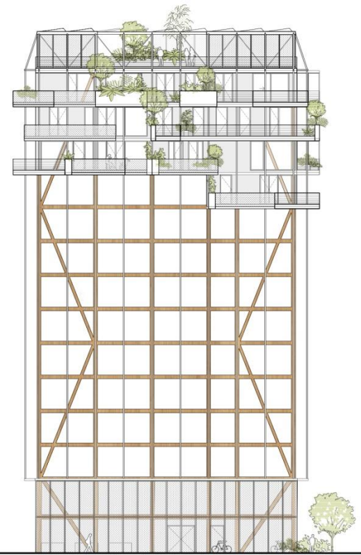
Façade Sud-Est
