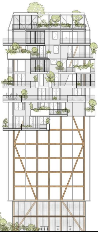
Façade Nord-Est
