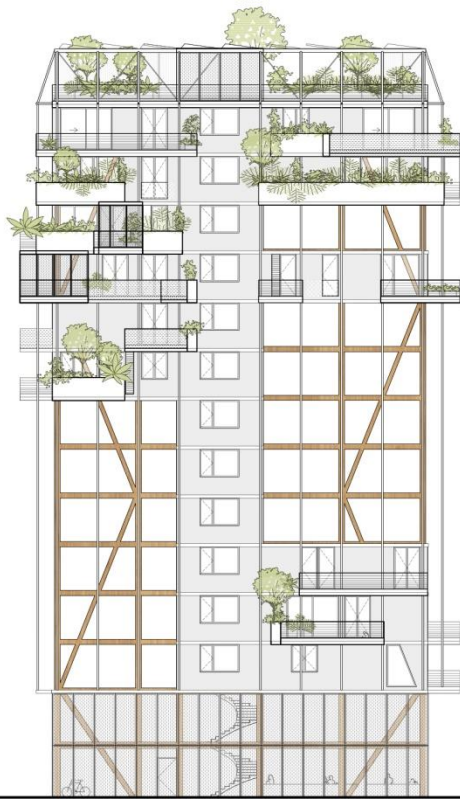
Façade Nord-Ouest
