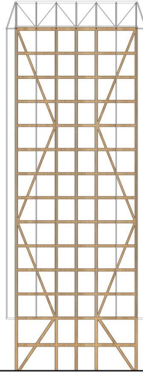
Façade Sud-Ouest
