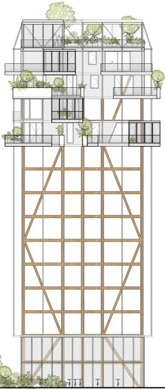
Façade Nord-Est
