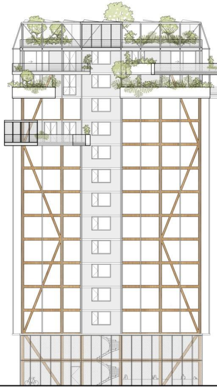
Façade Nord-Ouest
