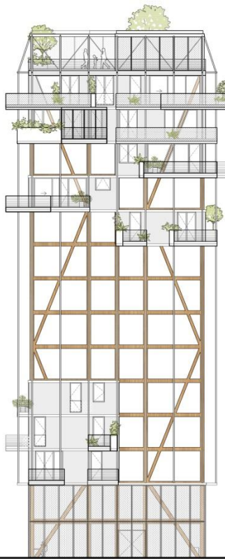
Façade Sud-Ouest
